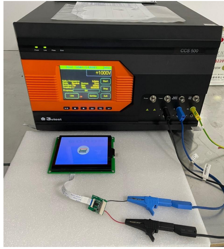
3.2 群脉冲测试图 EFT test
